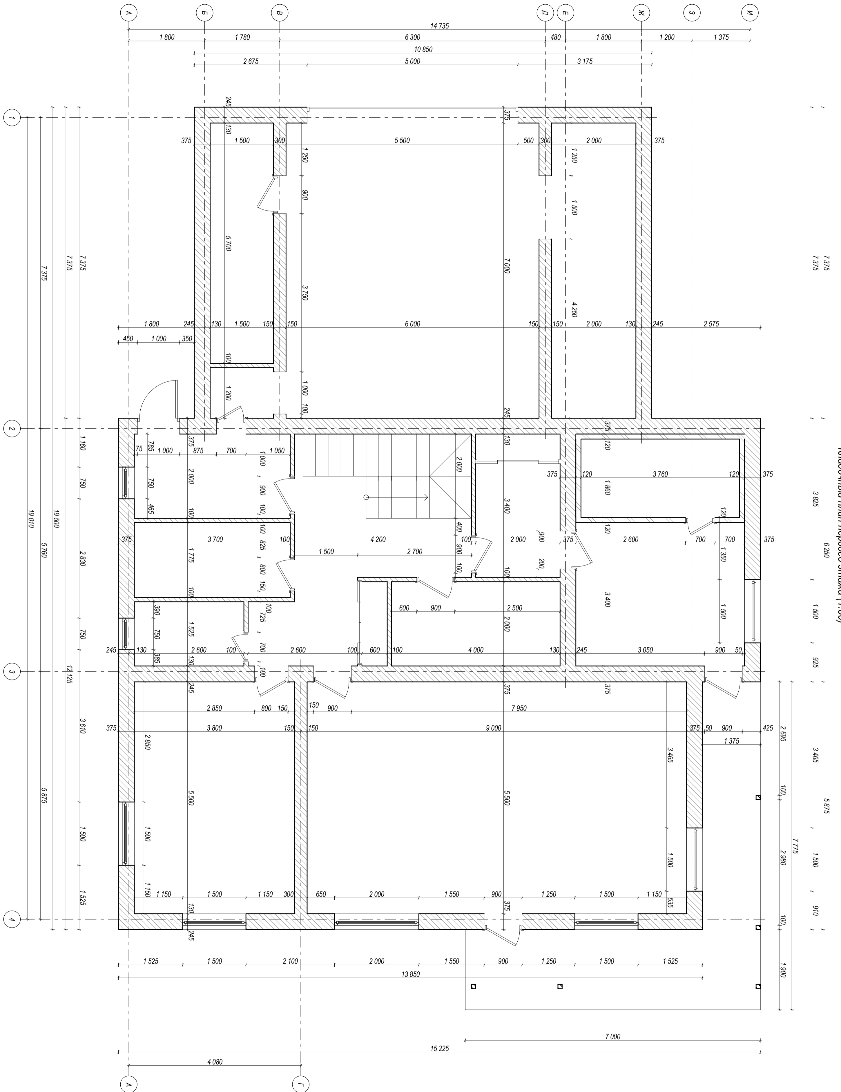
Кладочный план первого этажа (1:50)
